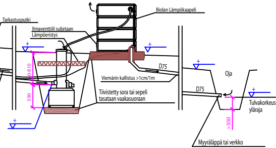
Harmaavesisuodatin 125
