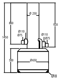
Pumppauskaivo
