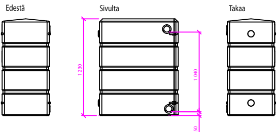
Harmaavesisuodatin 125
